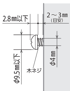
木ネジ取り付け状態
