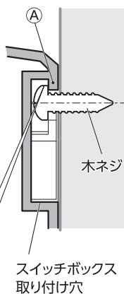
取り付け時の断面図
