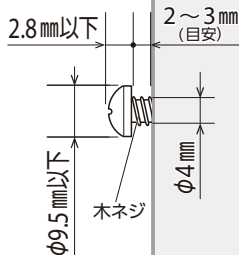
木ネジ取り付け状態
