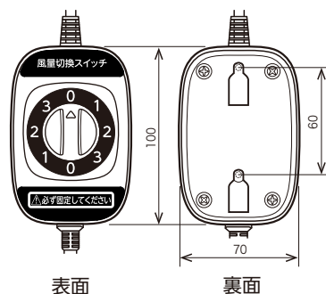
スイッチボックス取付寸法図 (単位:mm)
