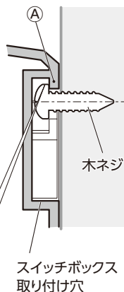
取り付け時の断面図
